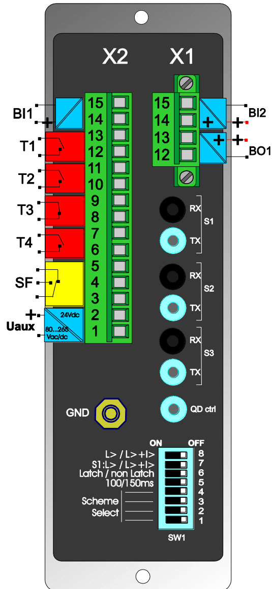
AQ102 connections.cdr
